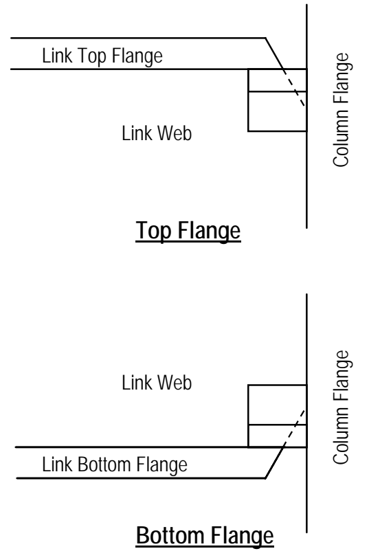
(d) NA-connections
