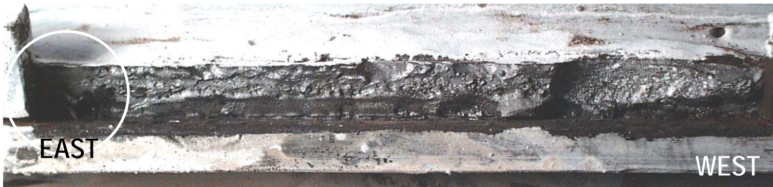
(d) PNM Top Flange (Not controlling failure mode)
