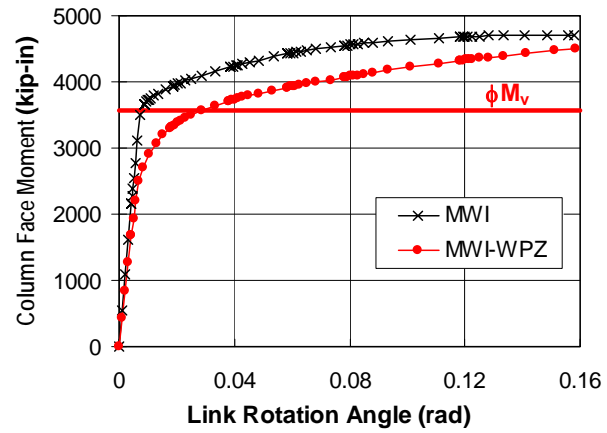
(d) Column Face Moment vs. Rotation Angle
