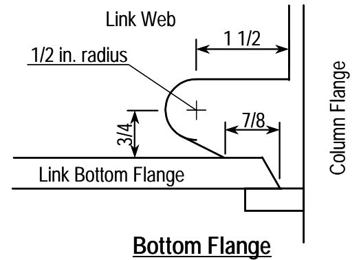
(b) MW-connections
